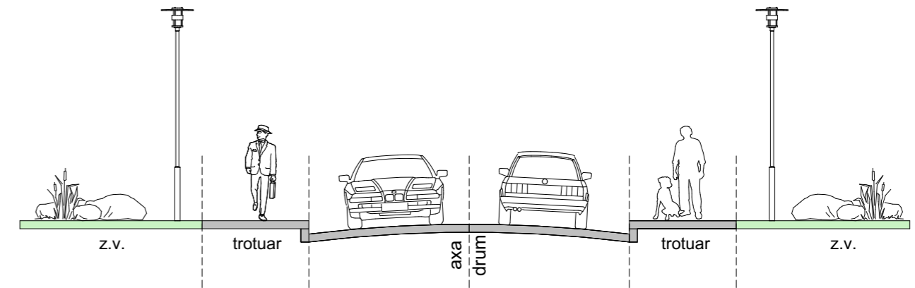
PROFIL TRANSVERSAL STRADA DE CATEGORIA A IV-A scara 1:100
